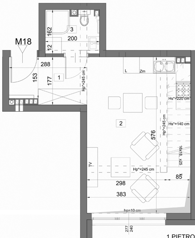
1 PIĘTRO
